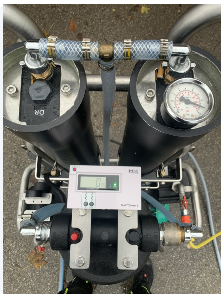
Mobile Reinwasseraufbereitung für die Glasreinigung.
