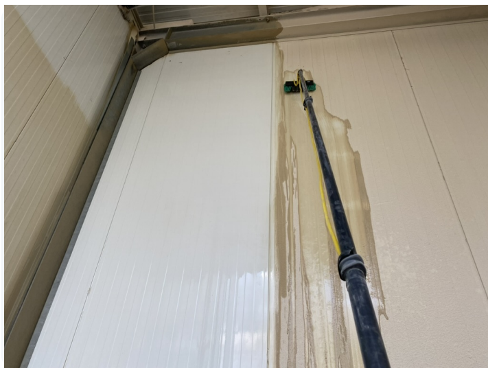
Reinigung einer Hallenwand mit wasserführender Bürste.
